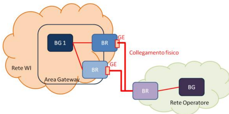
Figura 2: Modello architetturale d'interconnessione IP previsto da Vianova
