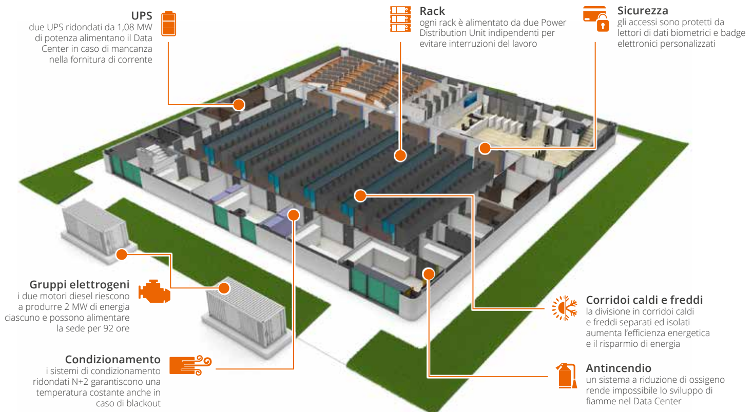
Layout del Data Center di Montacchiello (PI)
